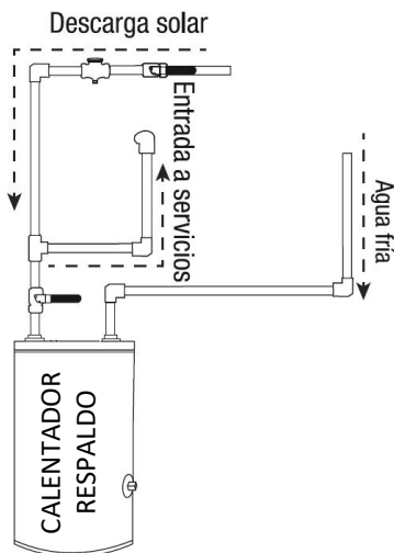
Función Calentador Solar
