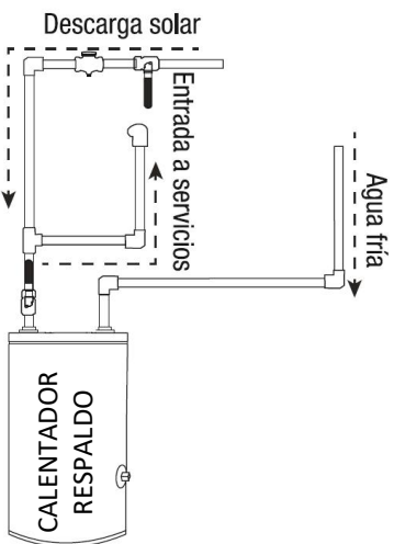
Función Calentador Respaldo
